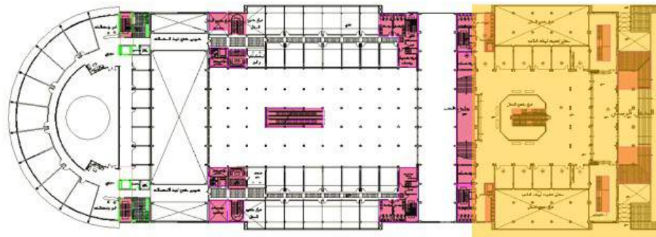
الجزء ( A ) الارضى
